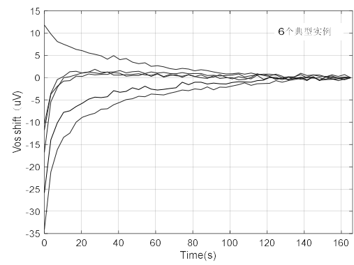
图8.8 失调电压偏移与时间的关系
