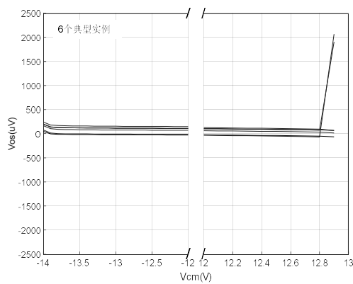
图8.9 失调电压与共模输入的关系
