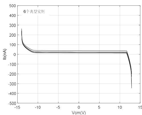
图8.13 偏置电流与共模输入的关系
