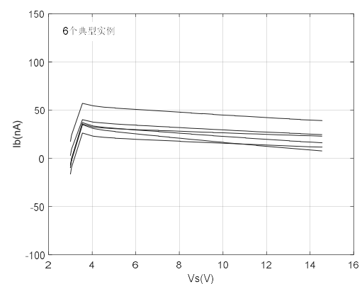
图8.14 偏置电流与供电电压的关系
