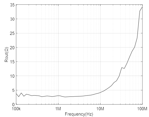
图8.22 开环输出阻抗与频率间的关系
