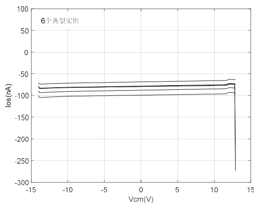
图8.11 失调电流与共模输入的关系
