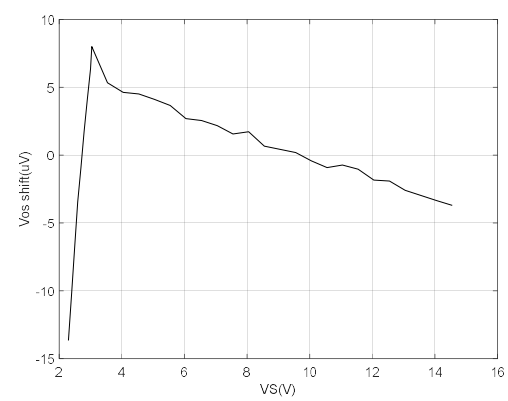
图8.10 失调电压偏移与供电电压的关系
