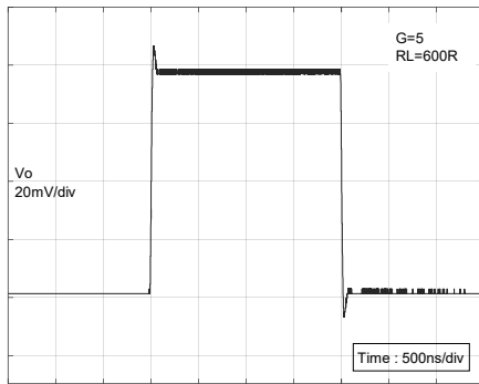
图8.15 小信号阶跃响应 (100 mVpp)
