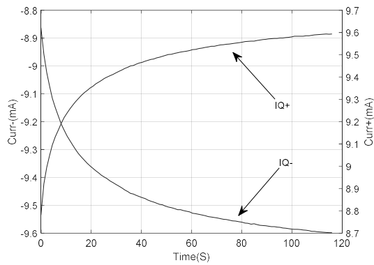
图8.7 静态电流与时间的关系
