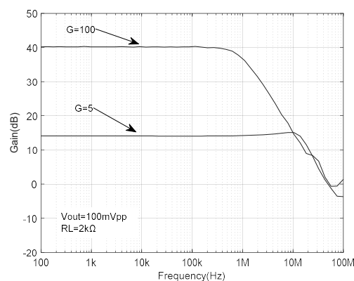
图8.6 闭环增益与频率间的关系
