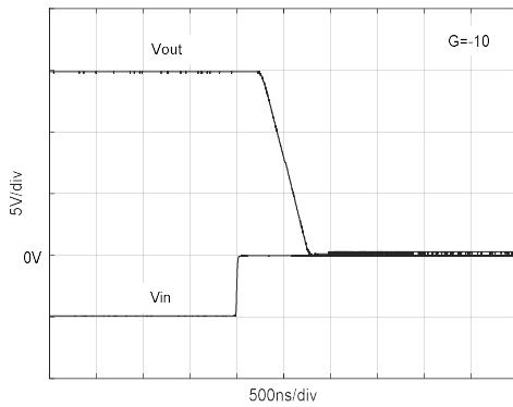
图8.17 正过载恢复时间
