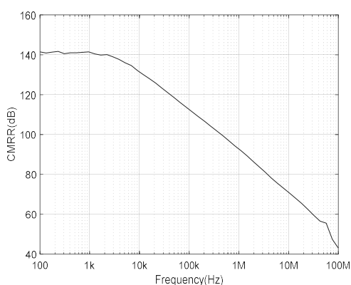
图8.5 共模抑制比
