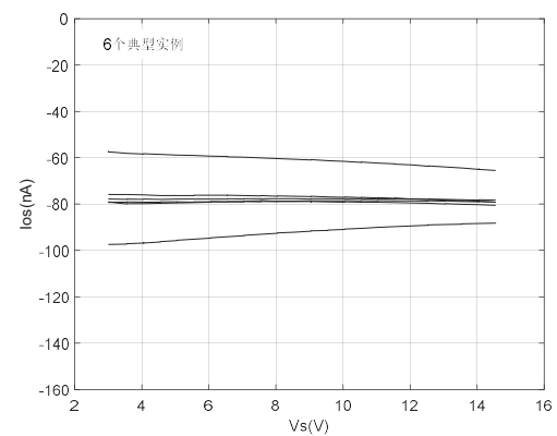
图8.12 失调电流与供电电压的关系
