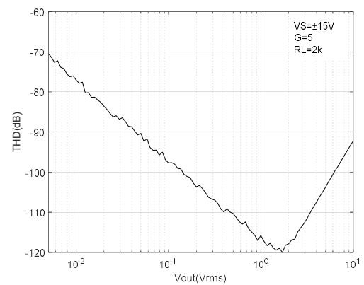
图8.20 输出摆幅和THD的关系
