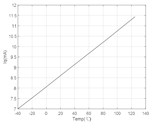
图8.19 静态电流与温度的关系
