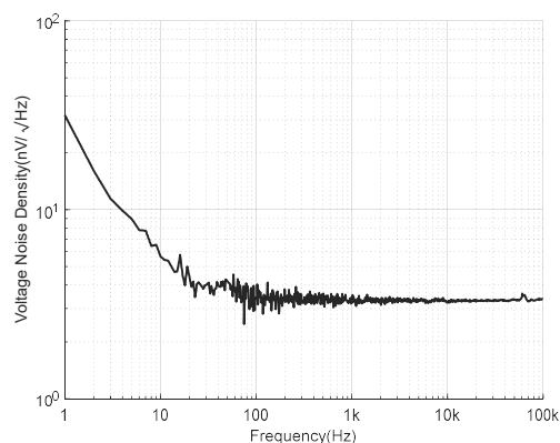
图8.2 电压噪声密度与频率的关系
