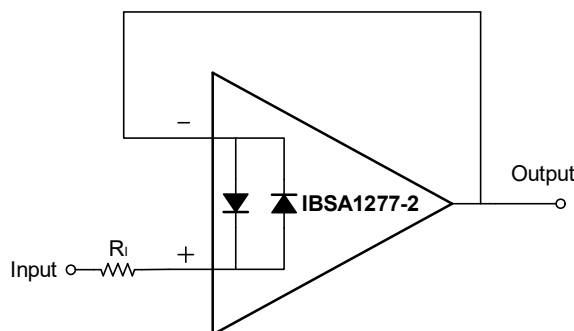
图10.2 输入保护示意图
