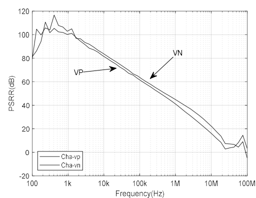
图8.4 电源抑制比
