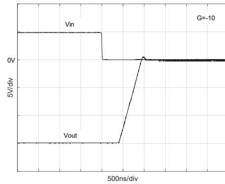
图8.18 负过载恢复时间
