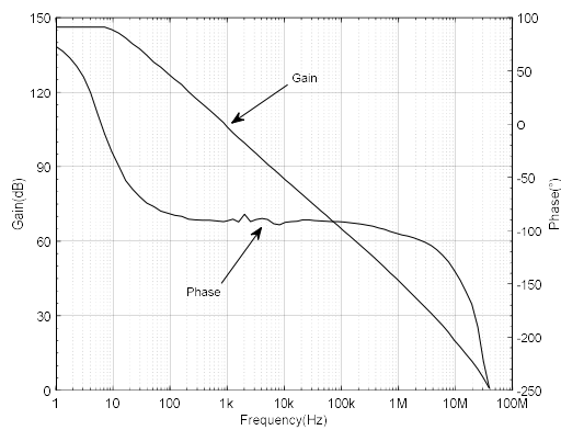
图8.21 开环增益和相位裕度
