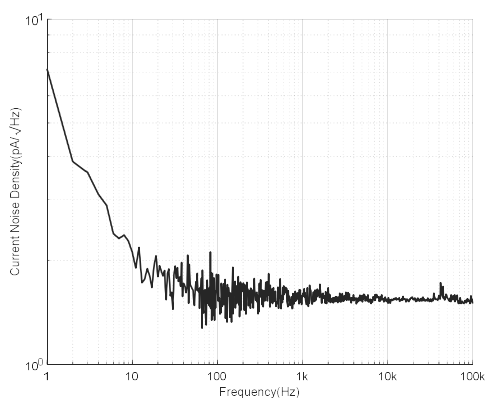
图8.3 电流噪声密度与频率的关系
